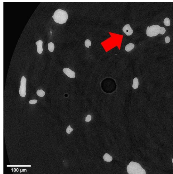
Fig.1 Al 系合金粉末の再構成処理像の例
