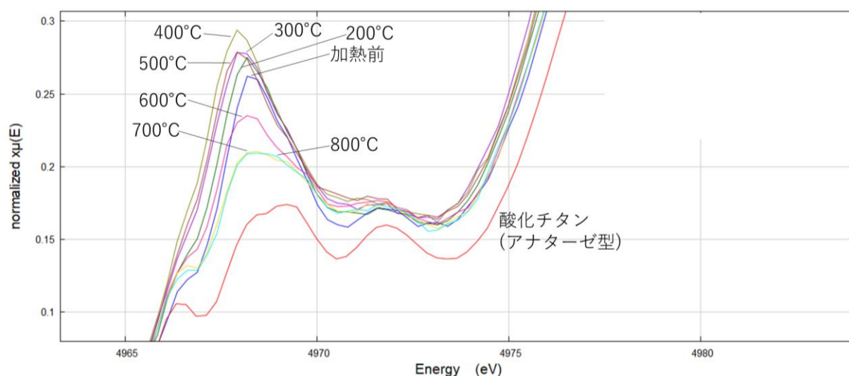
図 1. XAFS スペクトルの比較(He 雰囲気, 室温～800℃)
