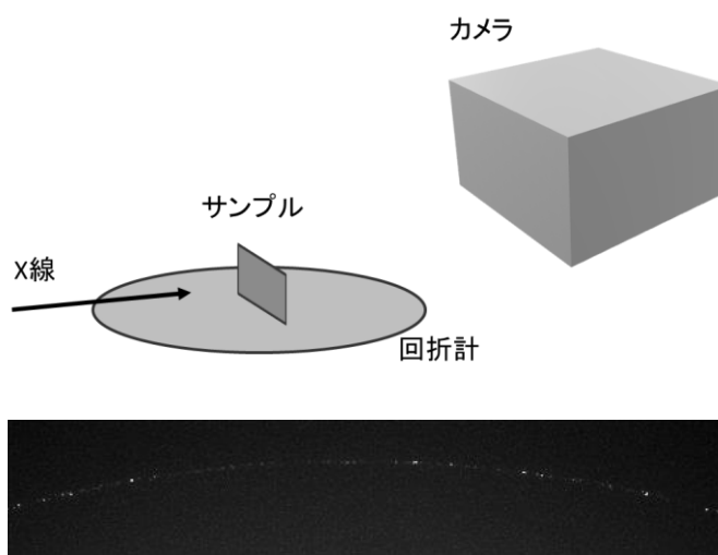
図1.測定の様式図（上）とデータ例（下） 2次元検出器を用いて、金結晶の回折点を観測し、 試料作製条件の検討を行った。
