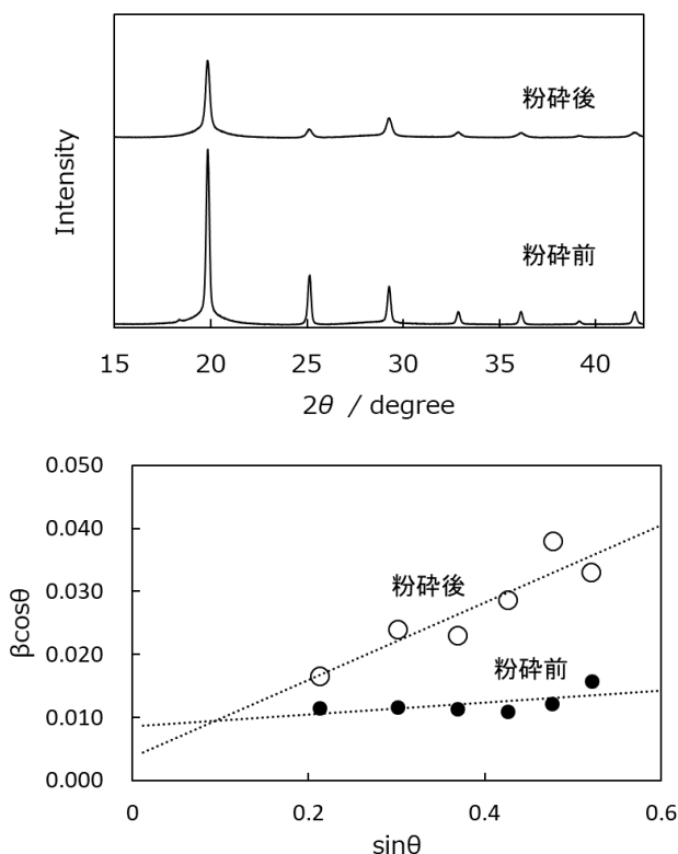
図 1 SR-XRD パターンおよび WH プロット
