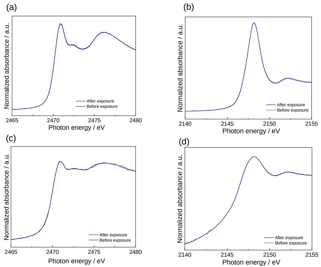
Fig. 1. 水蒸気暴露前後の \text{Li}_3\text{PS}_4 に対して、全電子収量法で測定した(a)S K-edge, (b)P K-edge XANES, 部分蛍光収量で測定した(c)S K-edge, (d)P K-edge XANES
