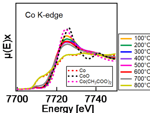
図 1 昇温中の Co 触媒のその場 XAFS スペクトル。
