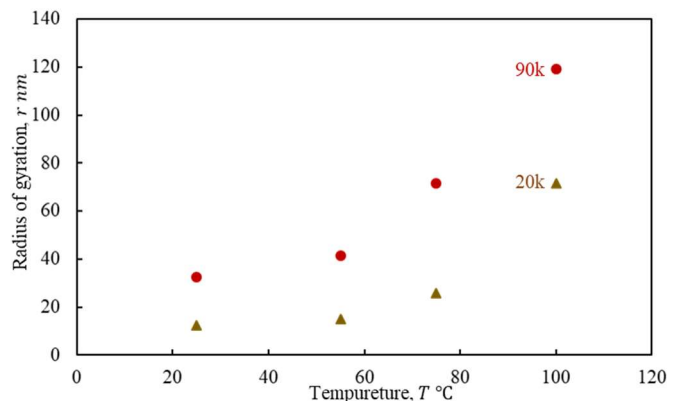
Fig. 1 鉱油中における PMA 系高分子の慣性半径の温度依存性
