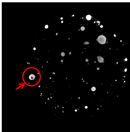
Fig.1 Cu 系合金粉末の X 線透過像を用いて再構成処理を行い得られた断面像の例
