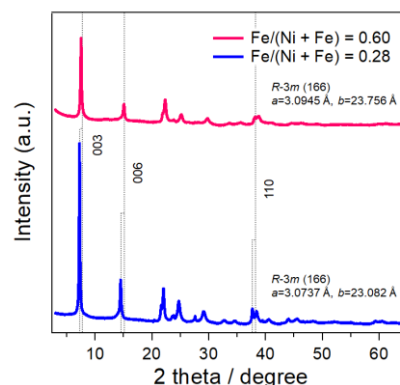
図. トポケミカル法で作製した Ni/Fe LDHs の S-XRPD パターンと指数付けの結果
