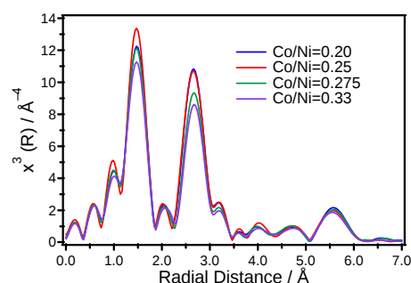
図. 種々の Co/Ni 比からなる LDHs の Co 周りの動径分布関数(RDF)
