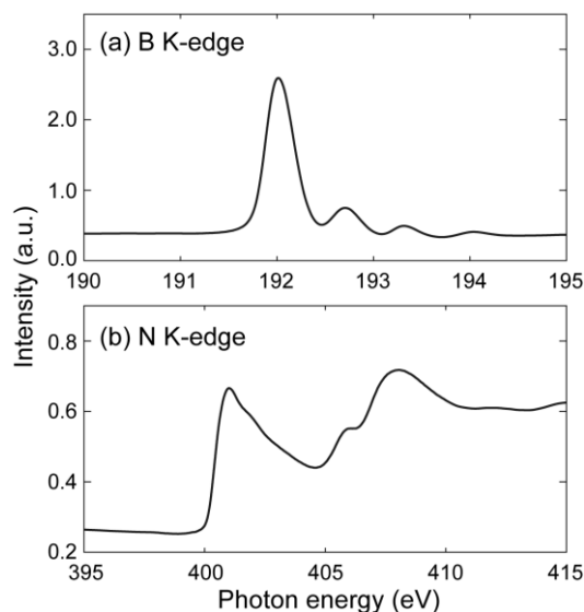
Fig.1 BCNO 薄膜の TEY-XAS : (a) B K-edge および (b) N K-edge.
