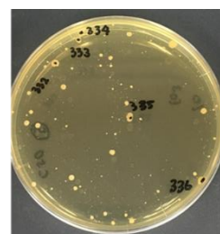
図 2 セルレニン耐性株 (照射 300 秒)
