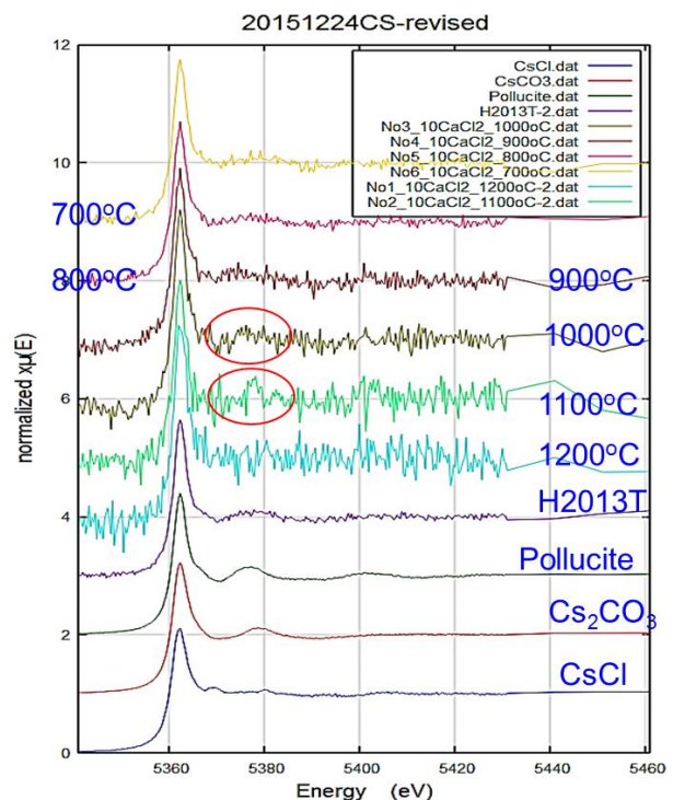
図1 各種試料中Csのスペクトル
