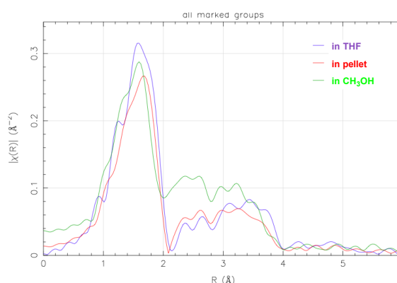
Fig.1 \text{CoCl}_2(\text{Naph-diPIM-dioxo-iPr}) の EXAFS スペクトル
